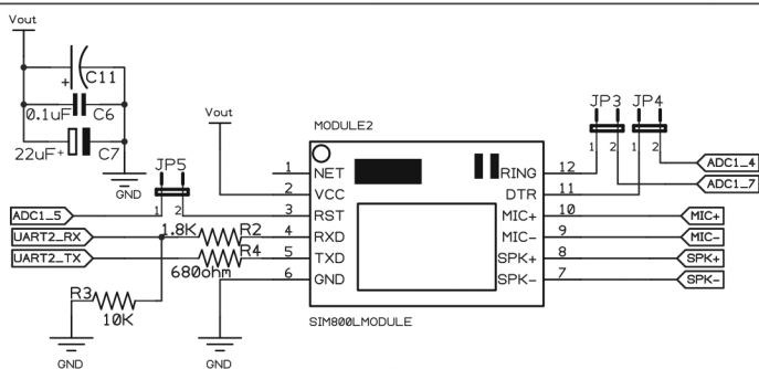
GSM Module
